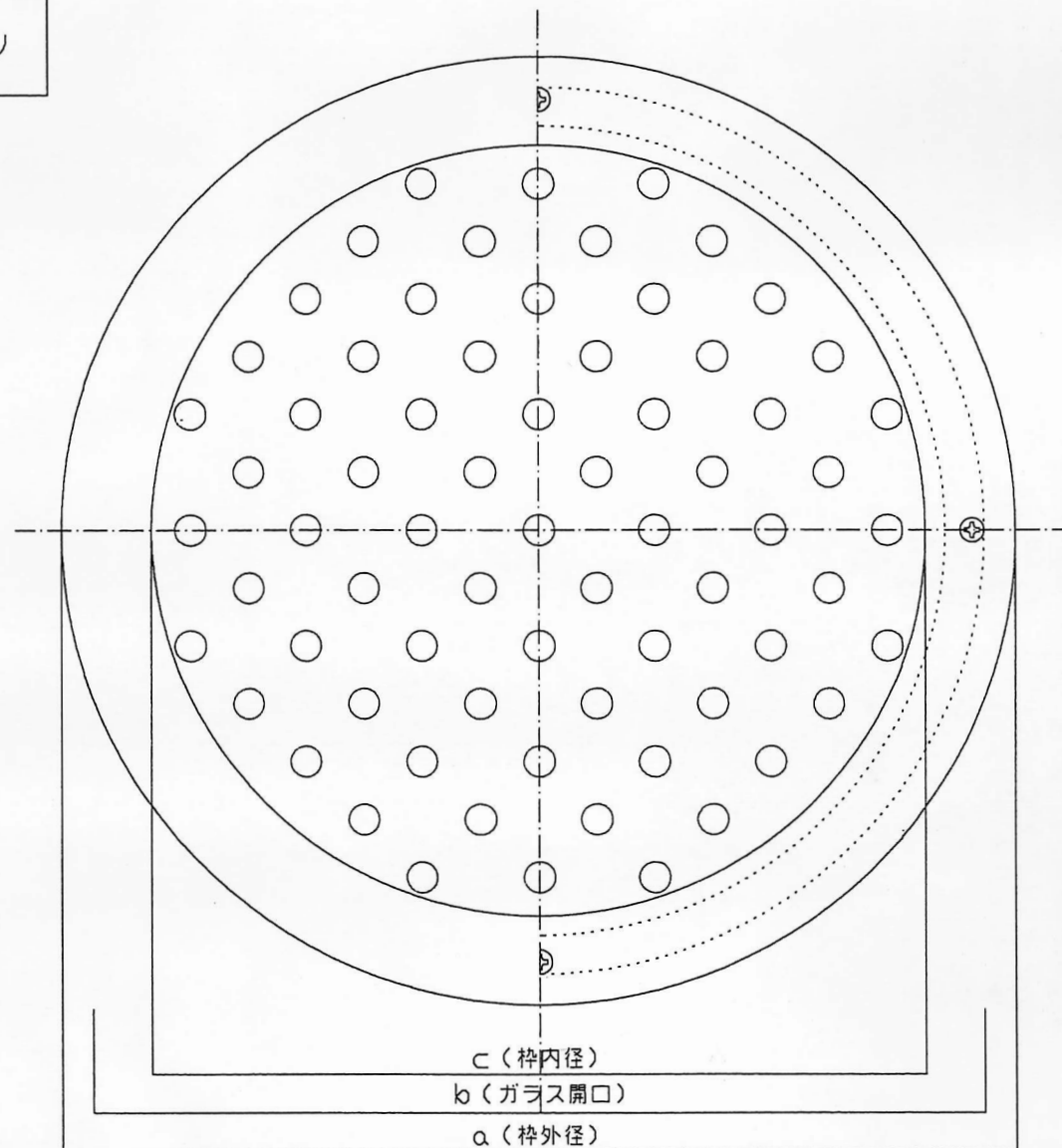
ビデオフォン (警察用 特殊) 姿図
