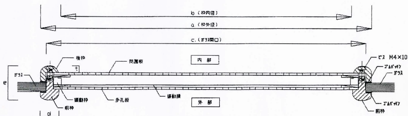
防護板付ビデオフォン規格
