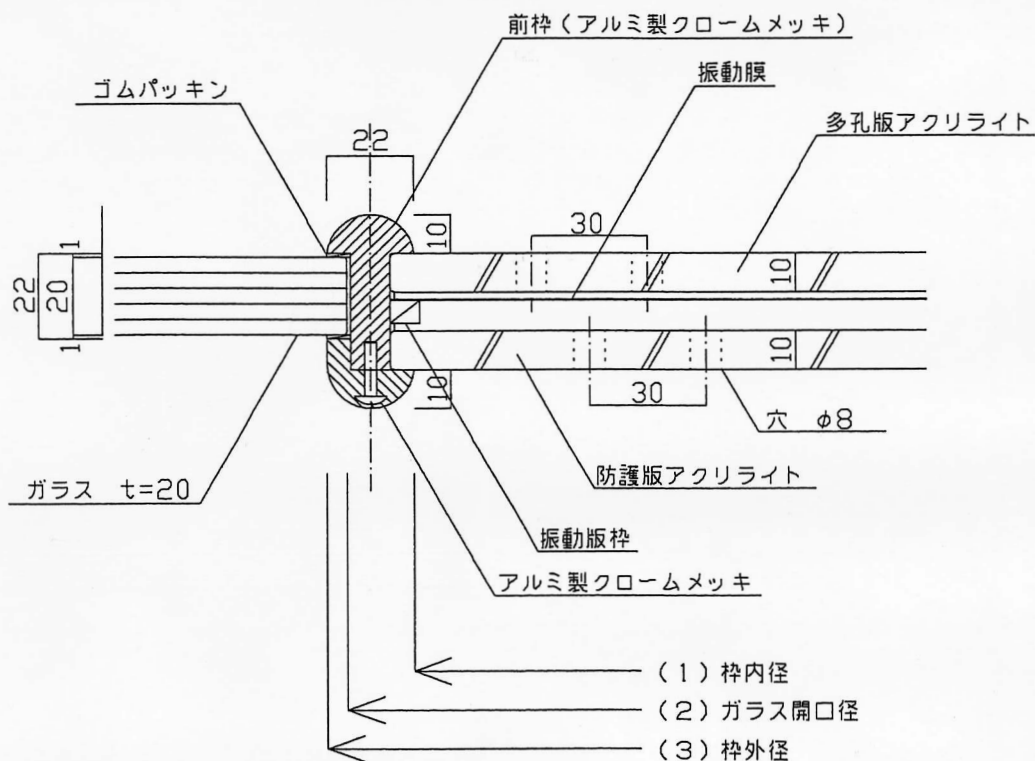
ビデオフォン (警察用 特殊) 断面図
